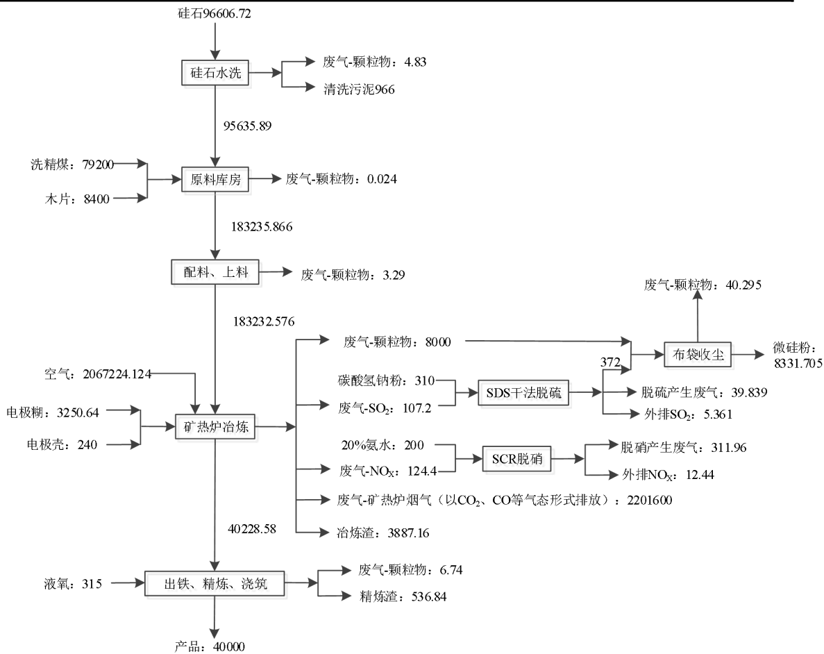
图 3.3-1 物料平衡图
