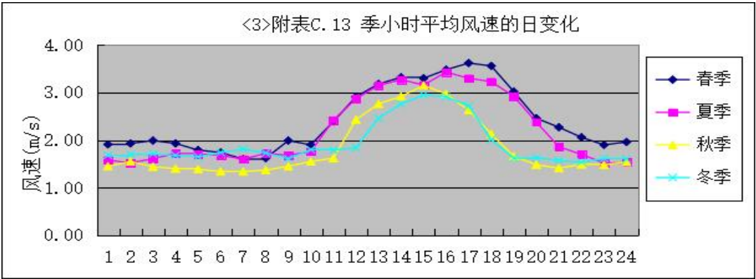
图 5.2-10 季小时平均风速日变化图
