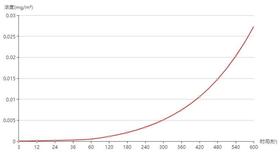
图 6.2-38 新城区初级中学浓度曲线图
