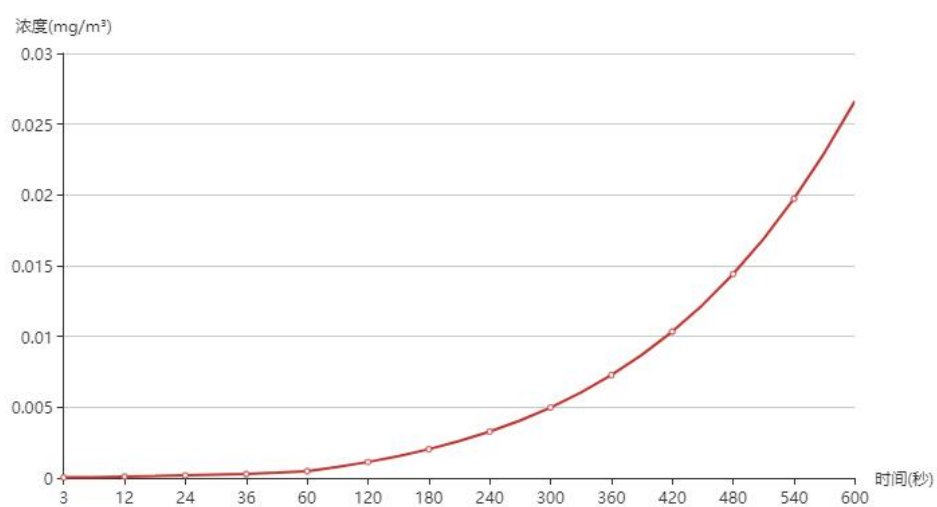
图 6.2-39 永登县第九中学浓度曲线图
