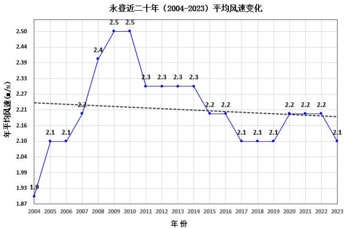
图 5.2-2 永登（2004-2023）年平均风速（单位：m/s）
