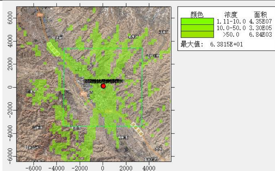
图 5.2-22 TSP24 小时质量浓度预测图
