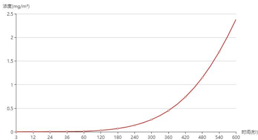
图 6.2-11 永登县农药管理局浓度曲线图
