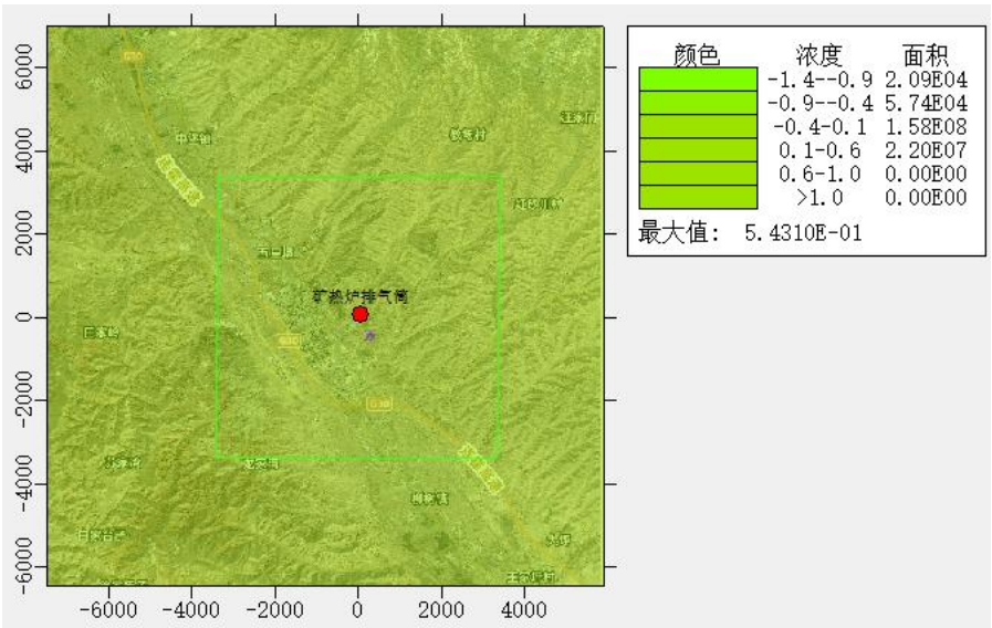
图 5.2-31 SO 2 年均质量浓度叠加预测图
