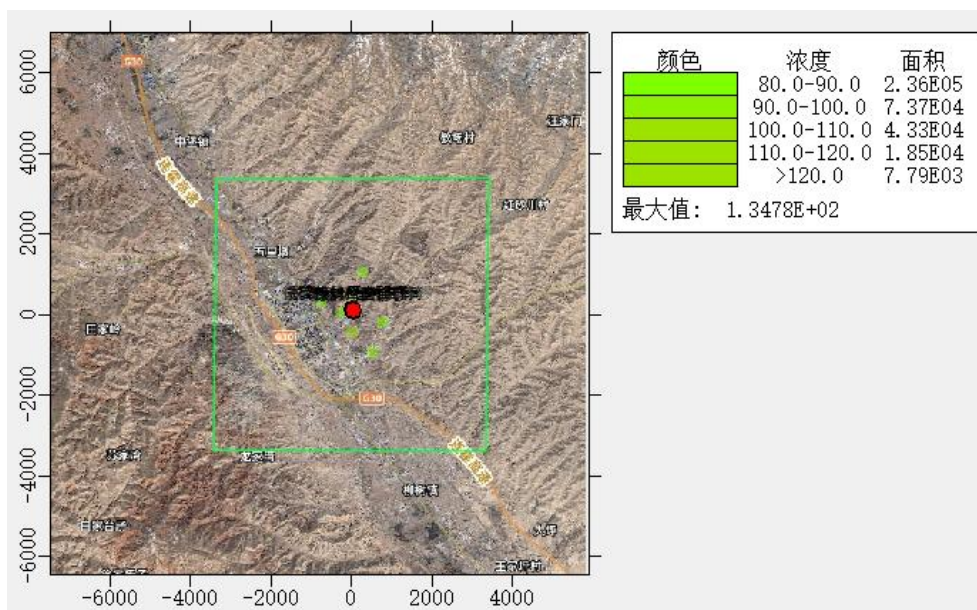
图 5.2-26 PM 10 24 小时质量浓度叠加预测图
