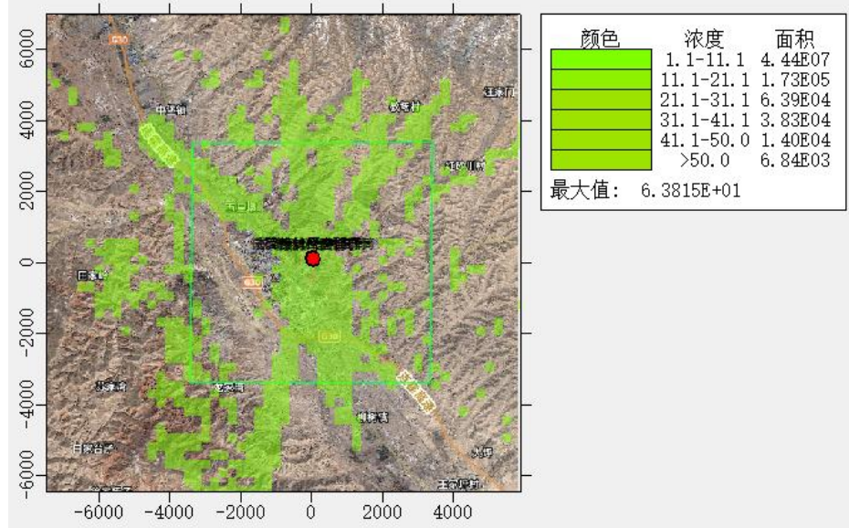
图 5.2-24 PM 10 24 小时质量浓度预测图
