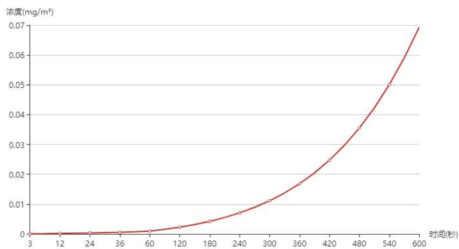
图 6.2-35 上坪浓度曲线图
