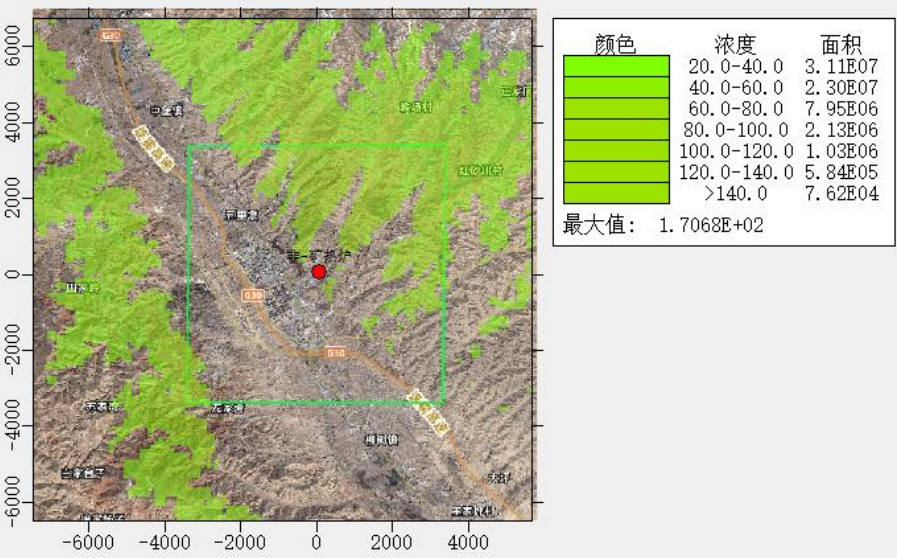
图 5.2-35 非正常工况 NO 2 1 小时质量浓度预测图
