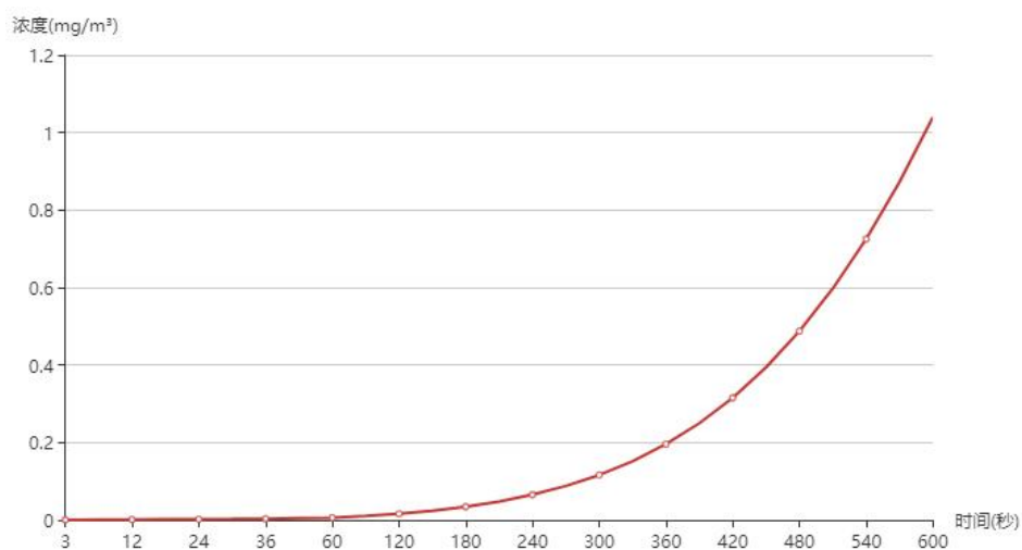
图 6.2-23 城关镇育才幼儿园浓度曲线图
