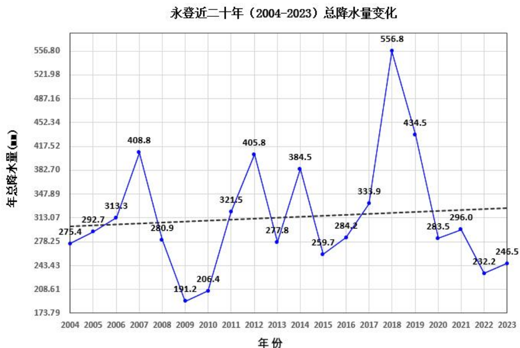
图 5.2-8 永登年平均降水量（单位：毫米，虚线为趋势线）
