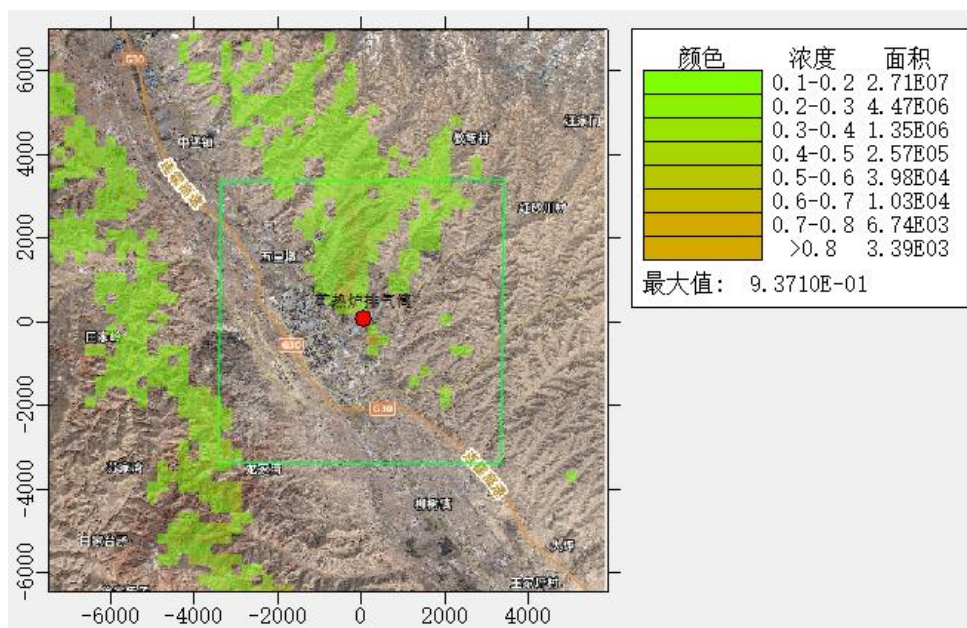
图 5.2-16 SO 2 年均质量浓度预测图
