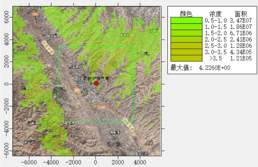
图 5.2-18 NO 2 日均质量浓度预测图
