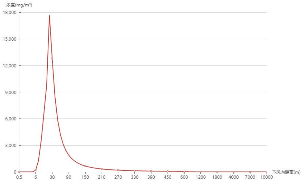
图 6.2-3 下风向不同距离处氨浓度曲线图
