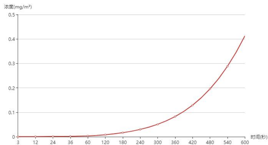
图 6.2-19 惠民花苑浓度曲线图
