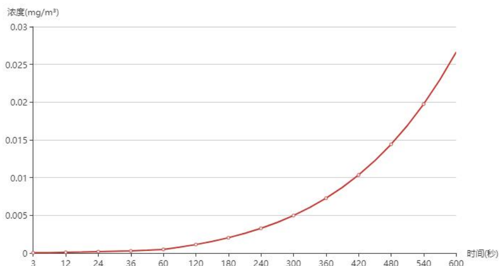
图 6.2-40 永登县高家湾小学浓度曲线图
