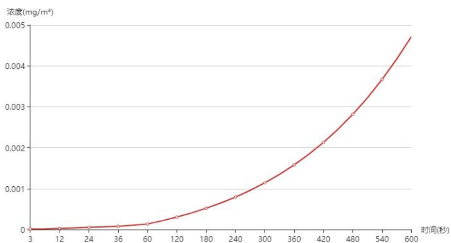
图 6.2-36 五渠村浓度曲线图
