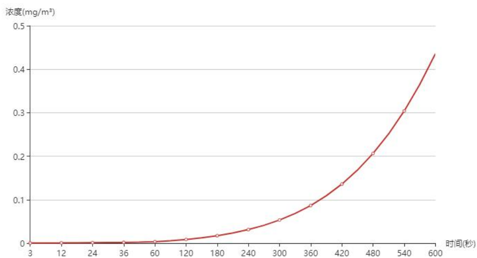
图 6.2-27 城关镇人民政府浓度曲线图
