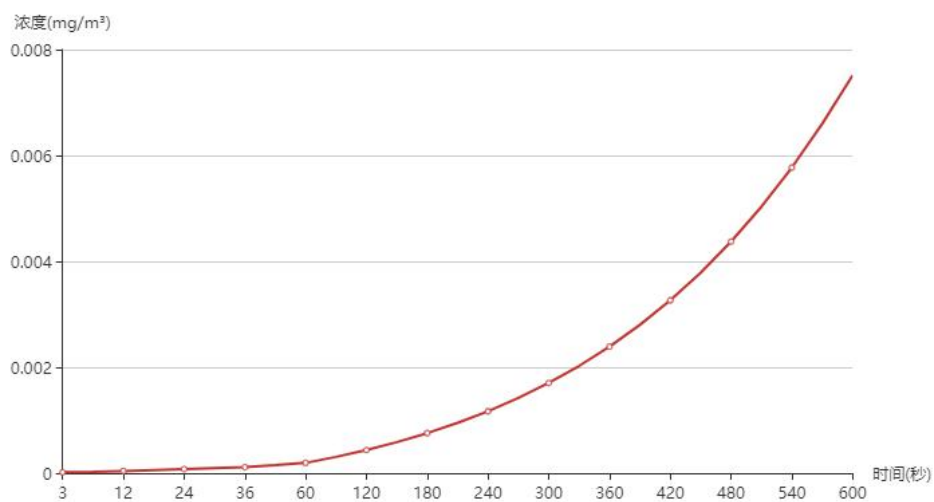
图 6.2-36 东湾浓度曲线图
