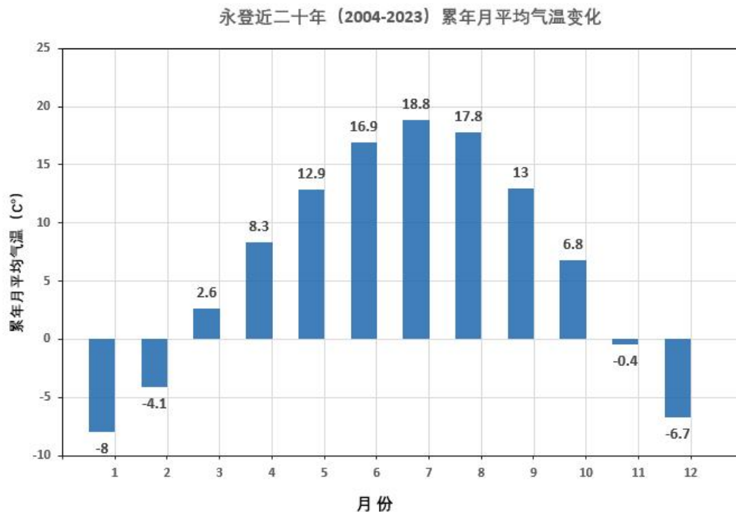
图 5.2-3 永登月平均气温（单位：°C）
