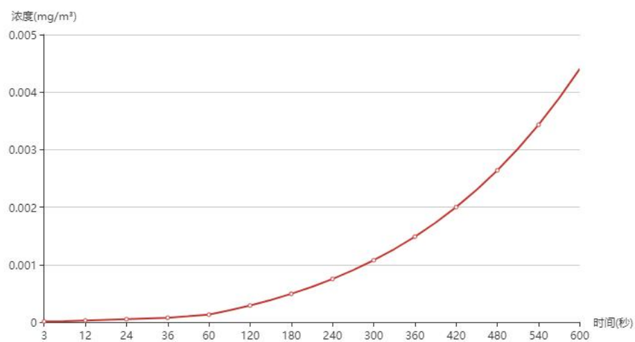
图 6.2-34 东坪浓度曲线图
