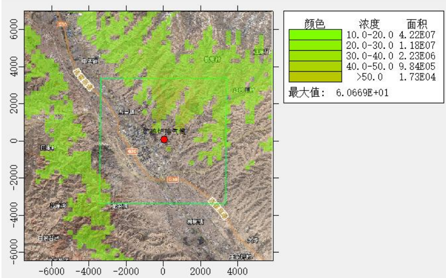
图 5.2-17 NO 2 1 小时质量浓度预测图
