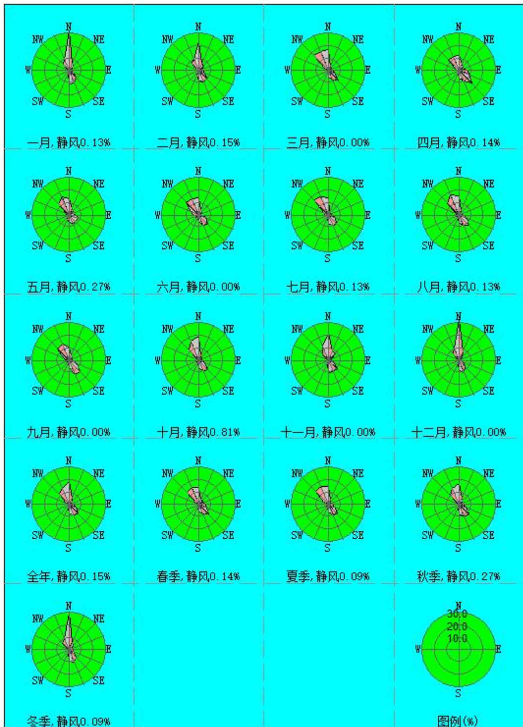
图 5.2-1 永登风向玫瑰 (2004-2023 年)
