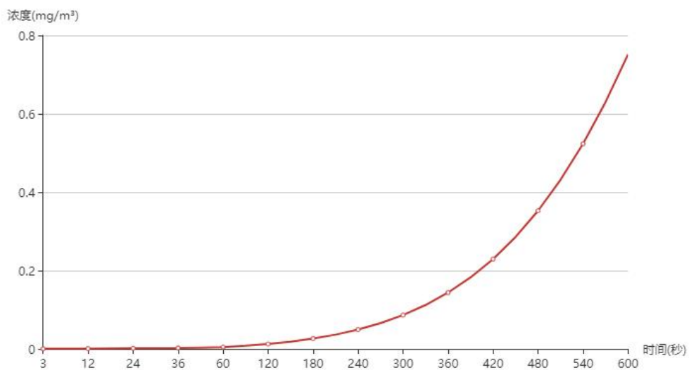
图 6.2-7 永登县第一中学浓度曲线图
