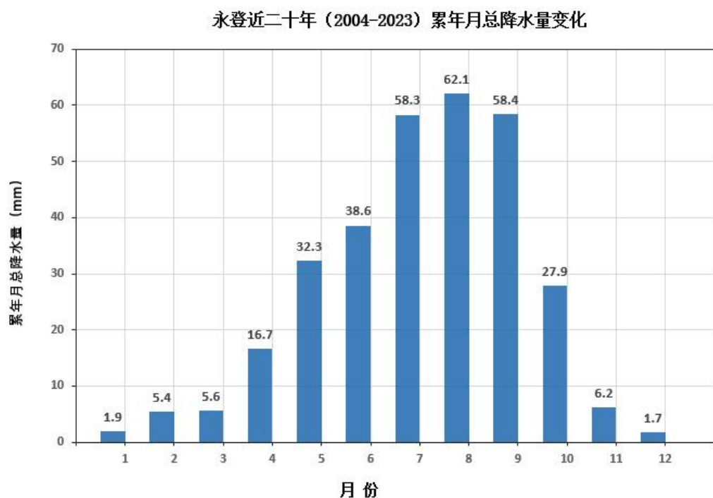
图 5.2-7 永登月平均降水量（单位：毫米）
