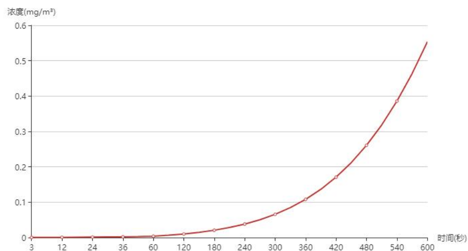
图 6.2-15 永登县新城区小学浓度曲线图
