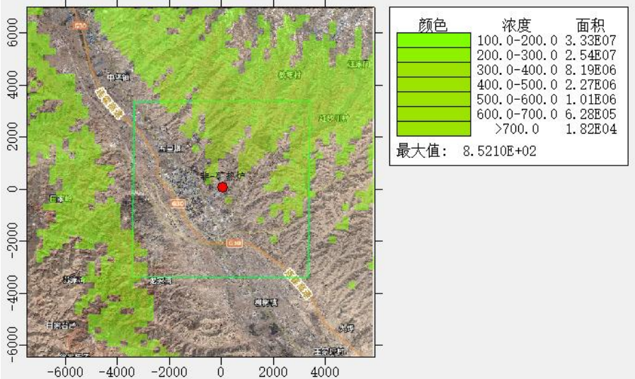
图 5.2-34 非正常工况 SO 2 1 小时质量浓度预测图
