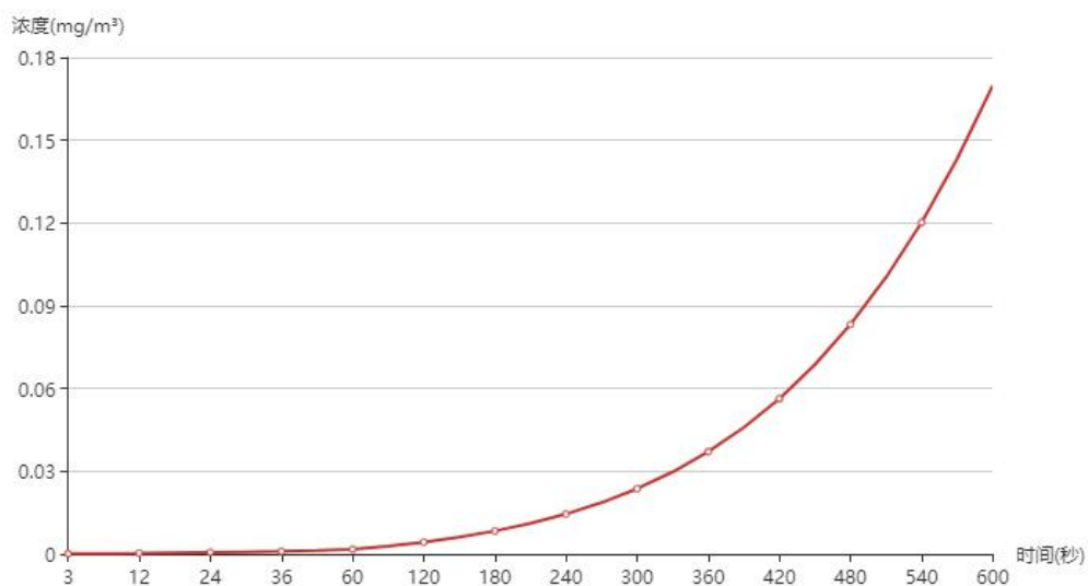
图 6.2-6 东街社区居委会浓度曲线图
