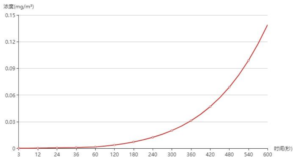
图 6.2-26 西街社区卫生服务站浓度曲线图
