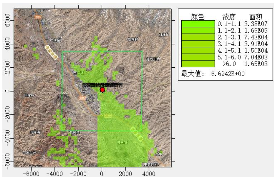
图 5.2-23 TSP 年均质量浓度预测图
