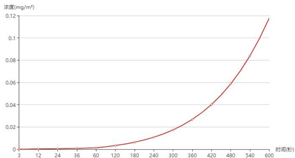
图 6.2-32 永登县第七中学浓度曲线图
