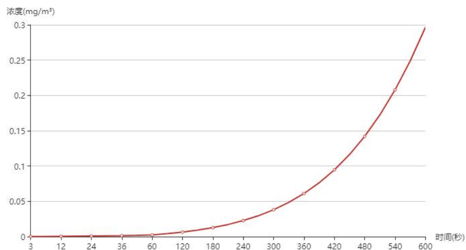
图 6.2-14 永登县满城小学浓度曲线图
