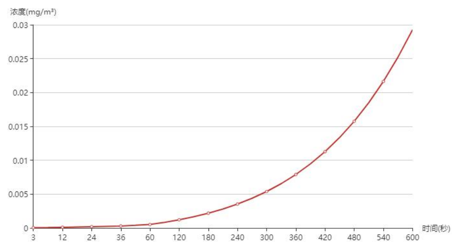
图 6.2-37 高家湾浓度曲线图
