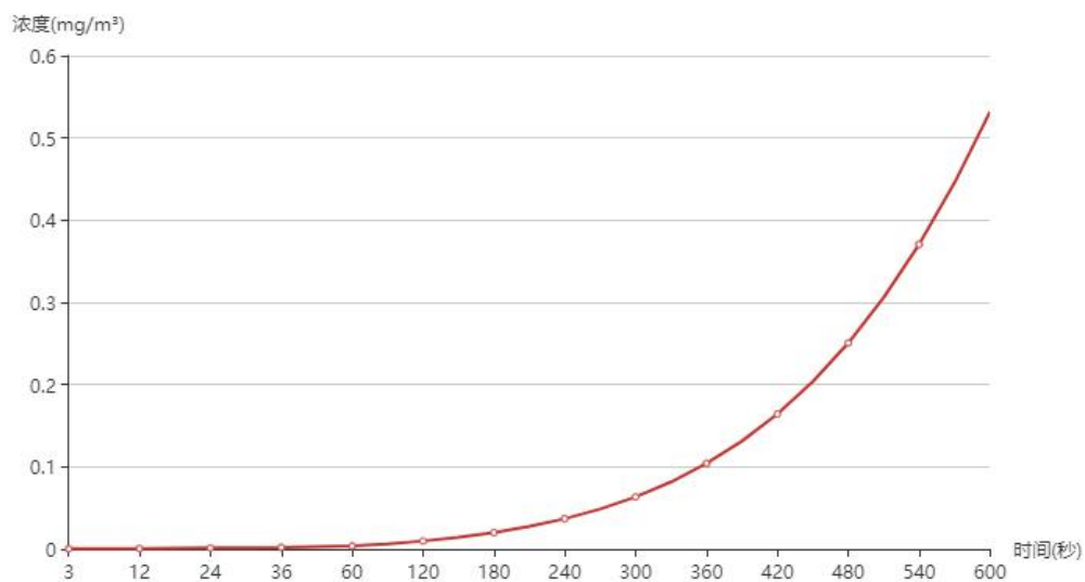
图 6.2-4 育才幼儿园浓度曲线图
