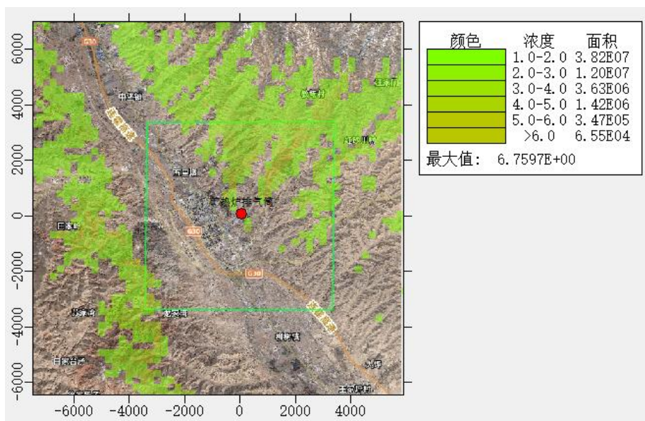
图 5.2-21 CO 日均质量浓度预测图
