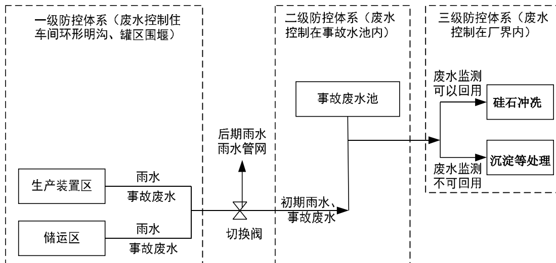
图 6.2-42 本项目三级防控体系及事故废水导排示意图
