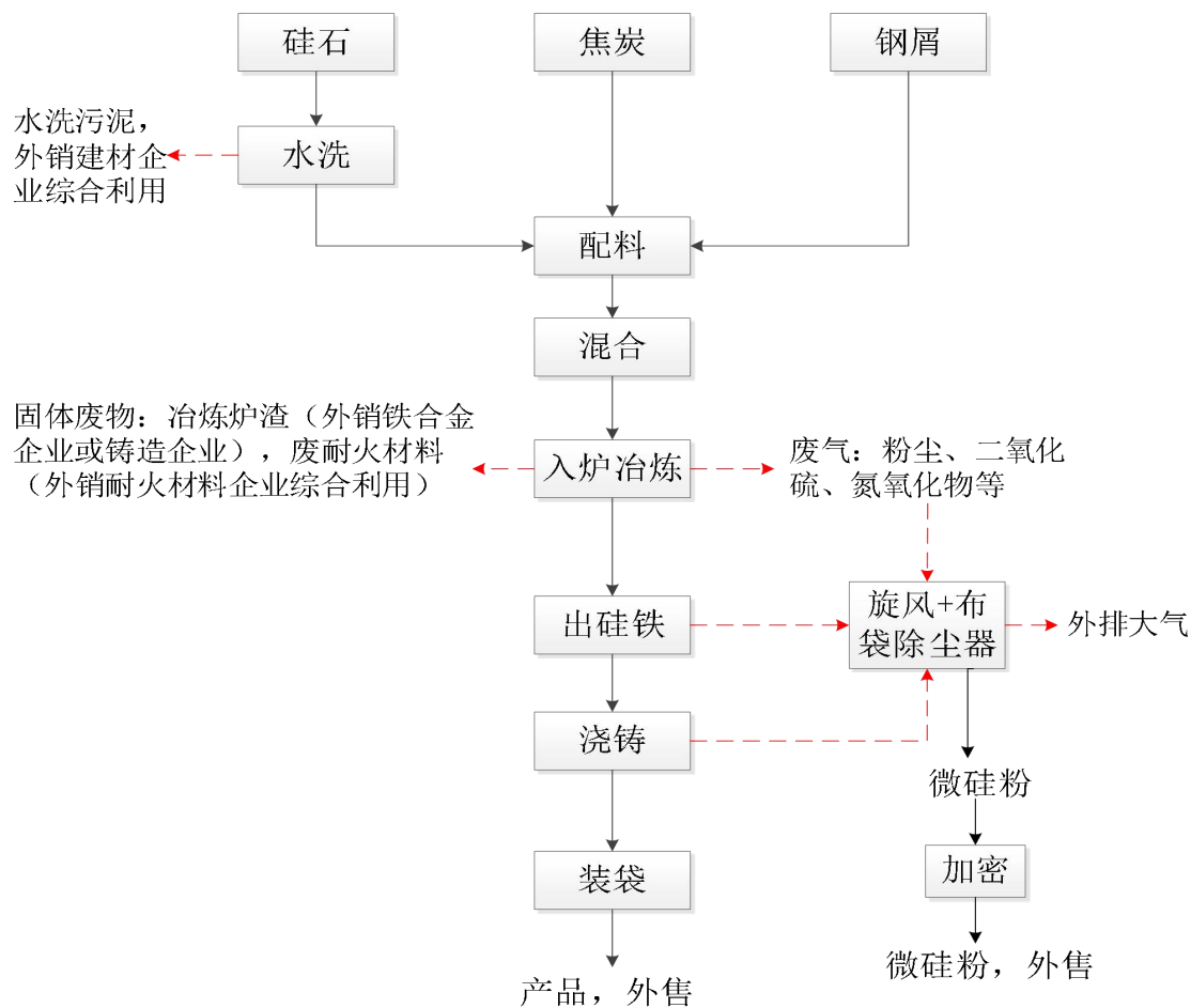
图 2.7-1 项目生产工艺流程及产污节点图
