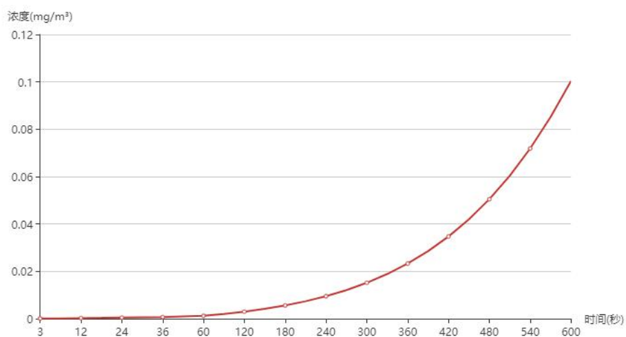
图 6.2-18 永登县种子管理局浓度曲线图
