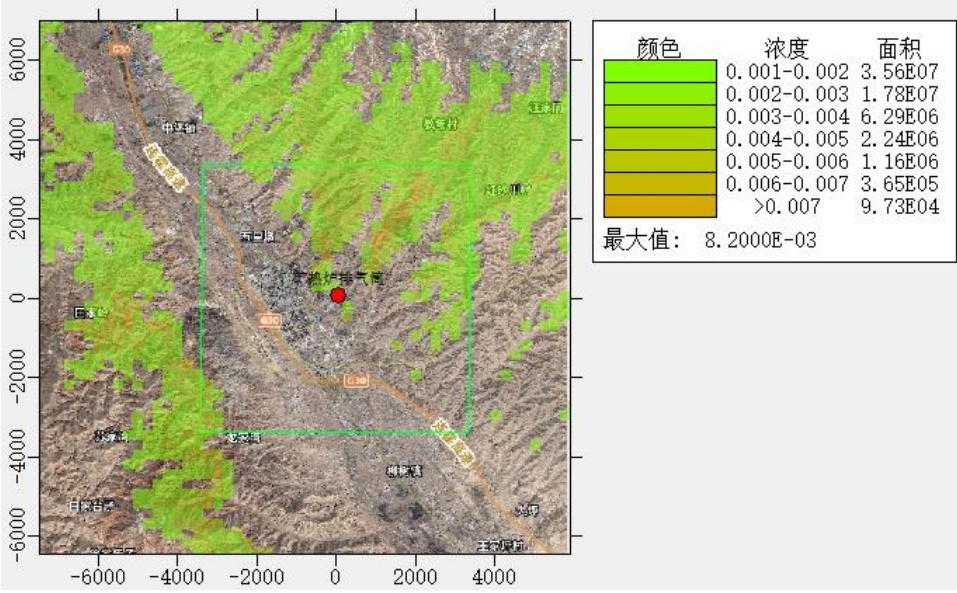
图 5.2-15 SO 2 日均质量浓度预测图
