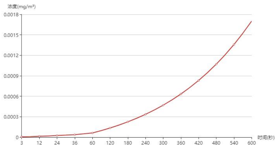
图 6.2-37 官庄浓度曲线图
