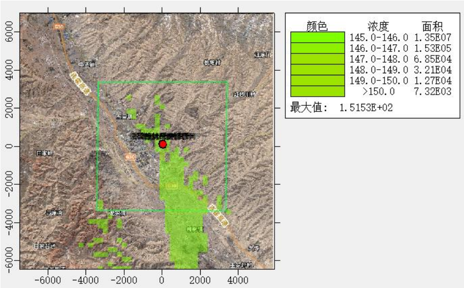
图 5.2-29 TSP 年均质量浓度叠加预测图
