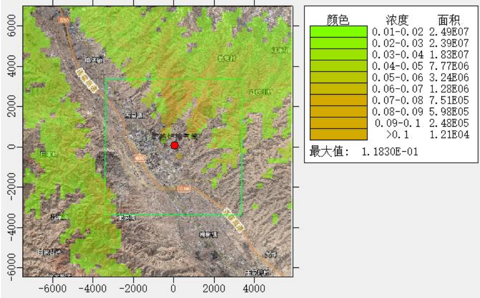
图 5.2-14 SO 2 1 小时质量浓度预测图
