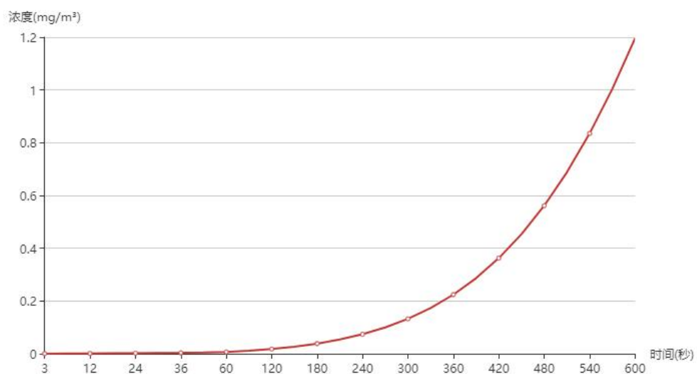
图 6.2-8 盛安医院浓度曲线图
