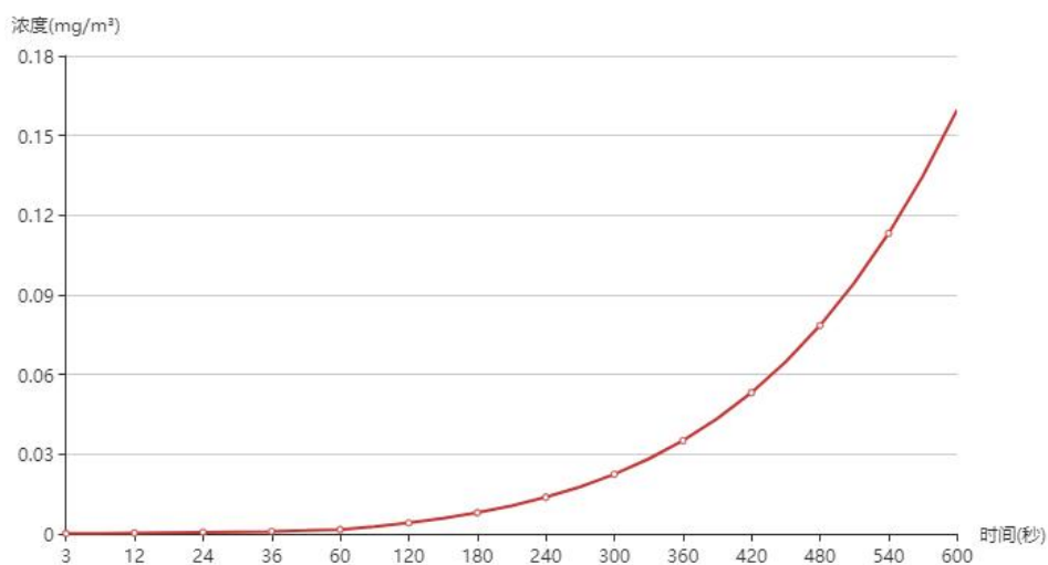
图 6.2-25 欣德嘉园浓度曲线图
