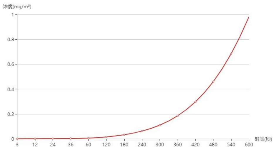
图 6.2-13 恒利天骄幼儿园浓度曲线图
