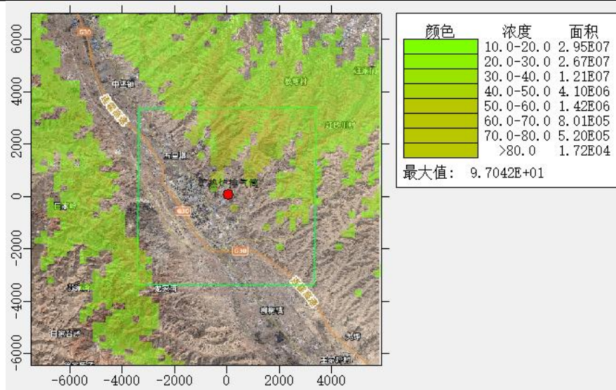
图 5.2-20 CO1 小时质量浓度预测图
