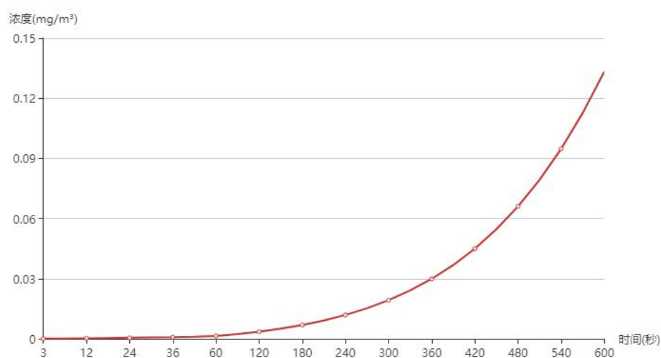
图 6.2-30 永登县三元堂医院浓度曲线图
