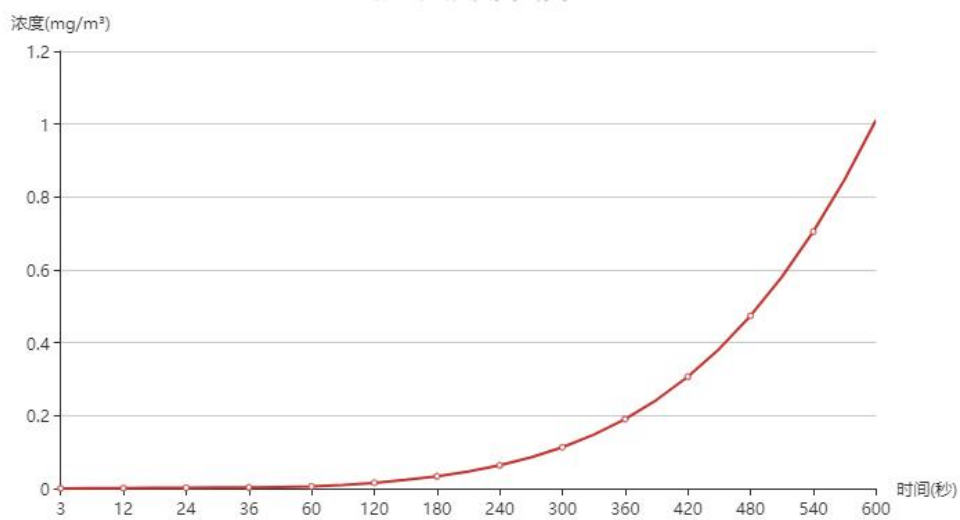
图 6.2-9 天成嘉园浓度曲线图
