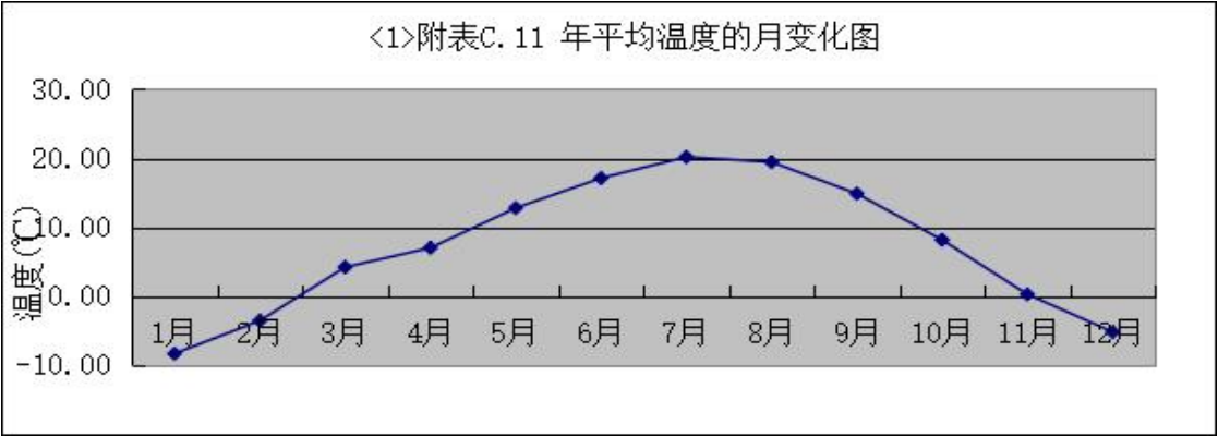
图 5.2-13 全年温度变化曲线图
