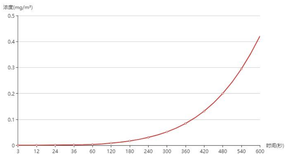
图 6.2-16 城关镇红乐园幼儿园浓度曲线图
