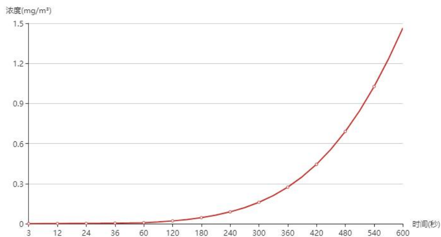
图 6.2-10 新泰嘉园浓度曲线图
