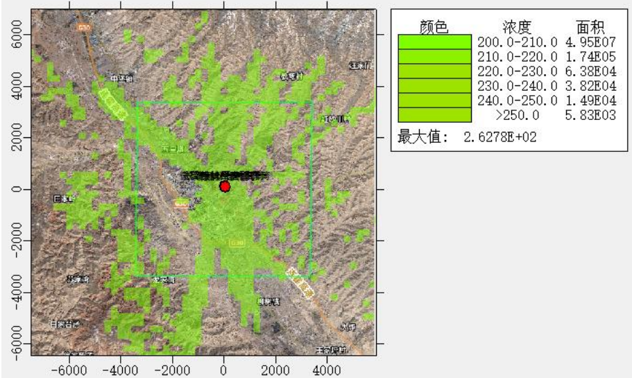
图 5.2-28 TSP24 小时质量浓度叠加预测图
