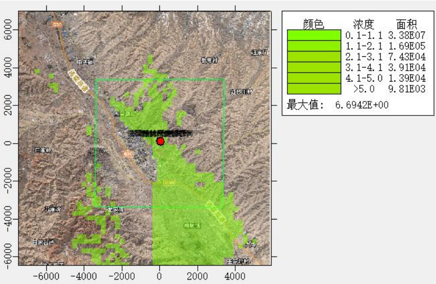
图 5.2-25 PM 10 年均质量浓度预测图
