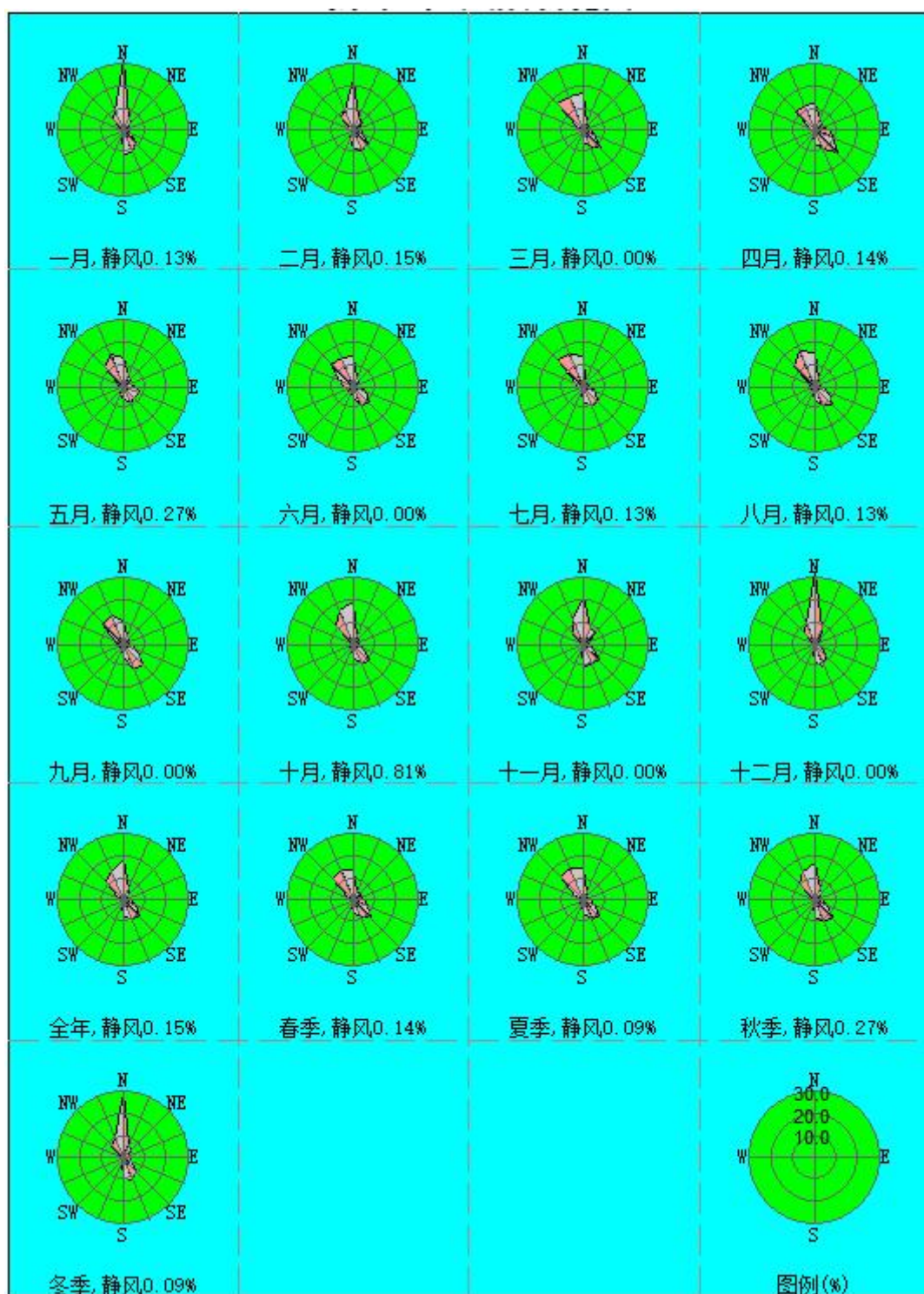
图 5.2-12 全年风向玫瑰图
