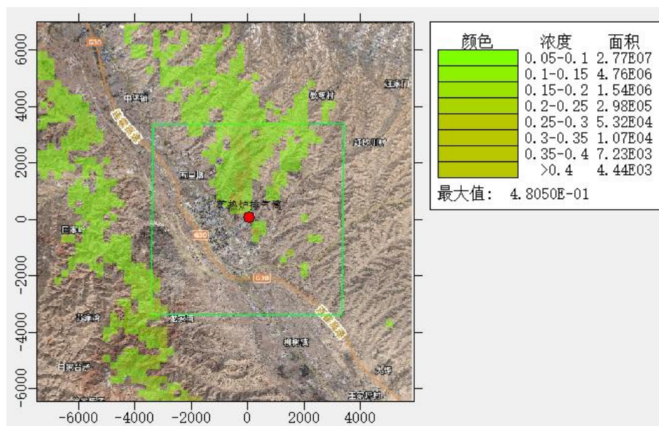
图 5.2-19 NO 2 年均质量浓度预测图
