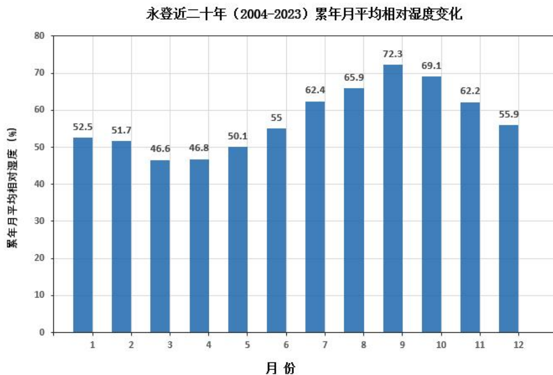
图 5.2-5 永登月平均相对湿度（纵轴为百分比）
