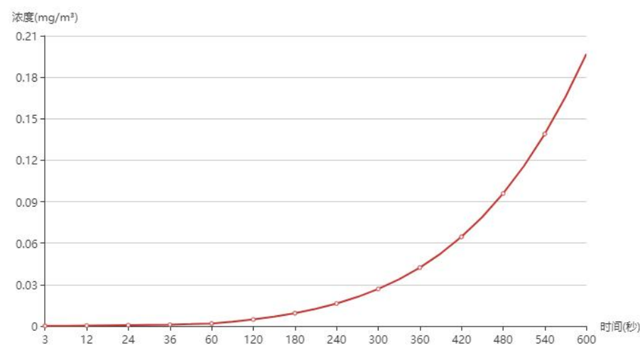
图 6.2-20 佳宁三期浓度曲线图
