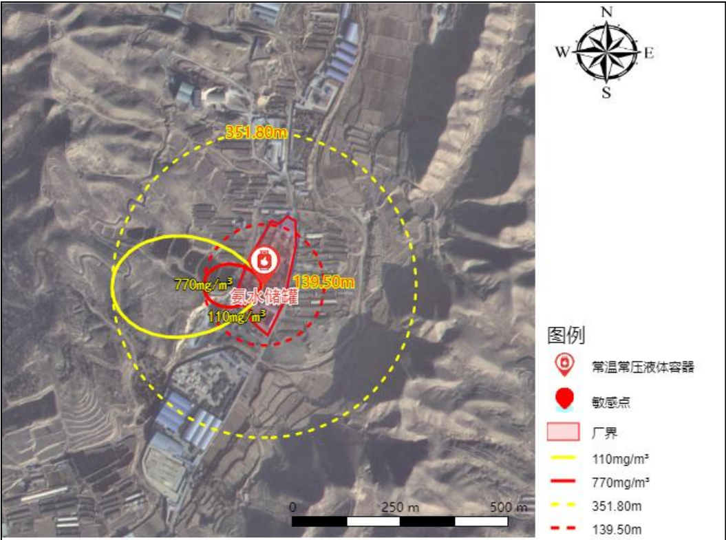
图 6.2-2 最不利气象条件下氨水储罐泄露产生氨气环境影响范围
