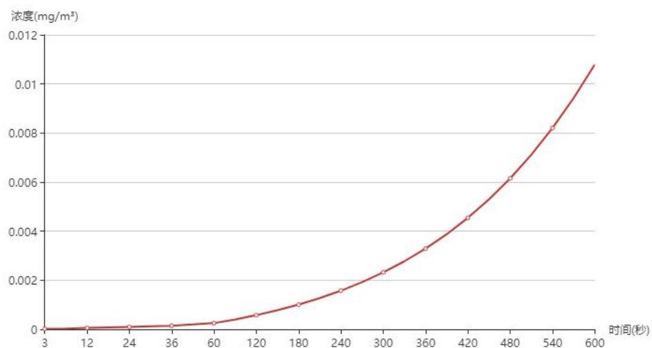
图 6.2-35 任家门浓度曲线图
