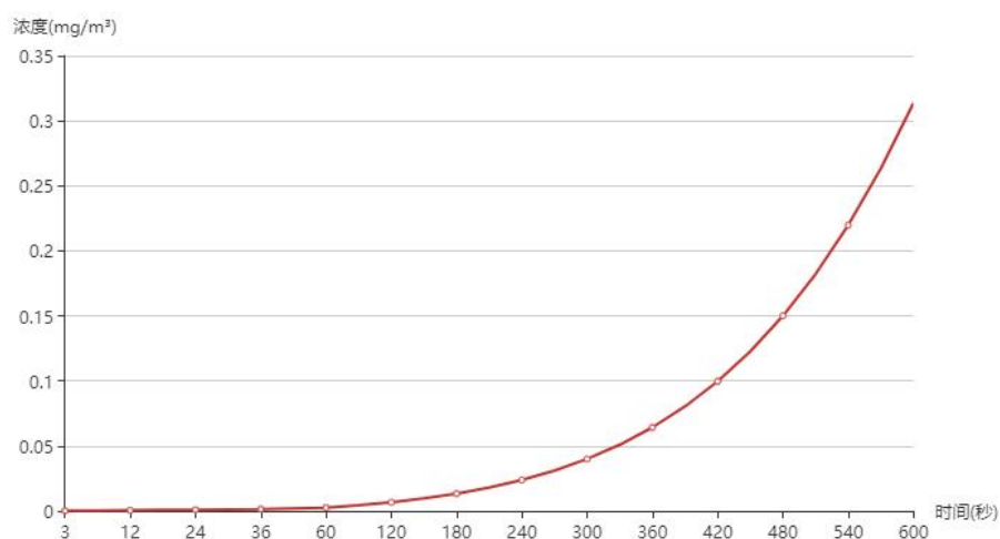
图 6.2-21 永登县人民医院浓度曲线图
