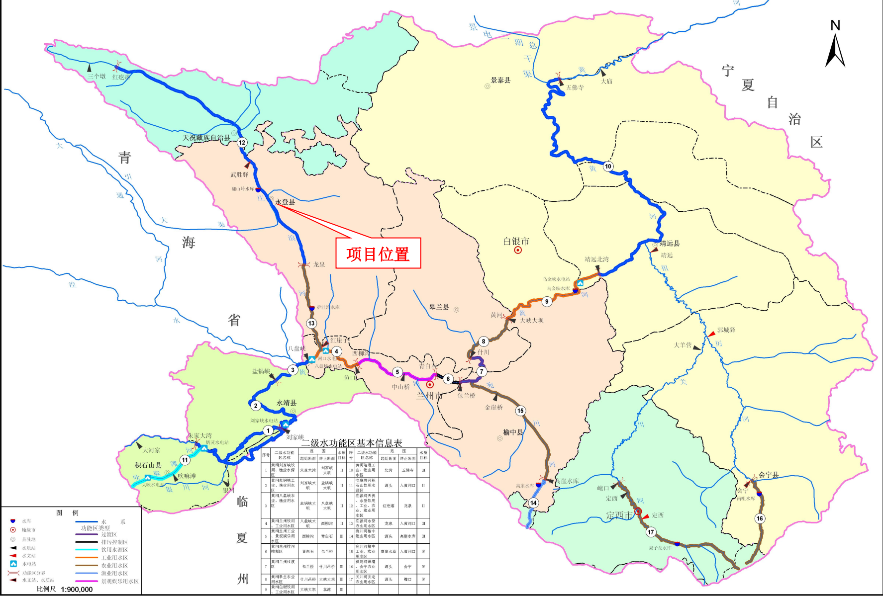
图 1.4-1 项目所在区域地表水功能区划图
