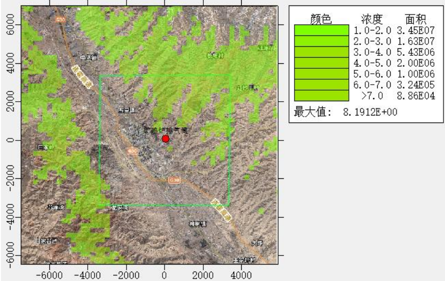
图 5.2-30 SO 2 24 小时质量浓度叠加预测图
