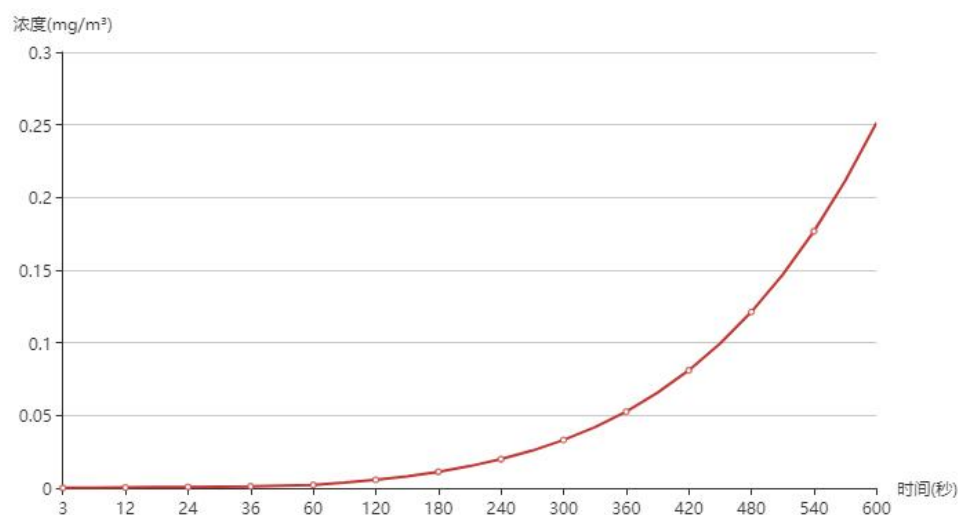
图 6.2-29 永登县人民政府浓度曲线图
