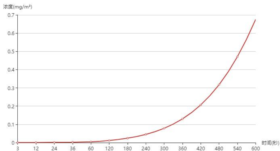
图 6.2-12 永登县盐务局浓度曲线图
