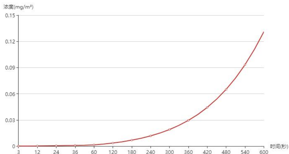
图 6.2-31 永登县龙岗小学浓度曲线图
