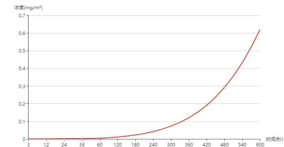
图 6.2-22 永登县第八中学浓度曲线图
