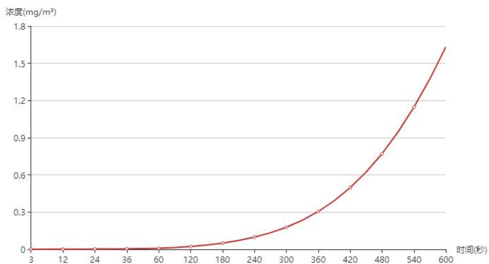
图 6.2-5 农机厂家属院浓度曲线图
