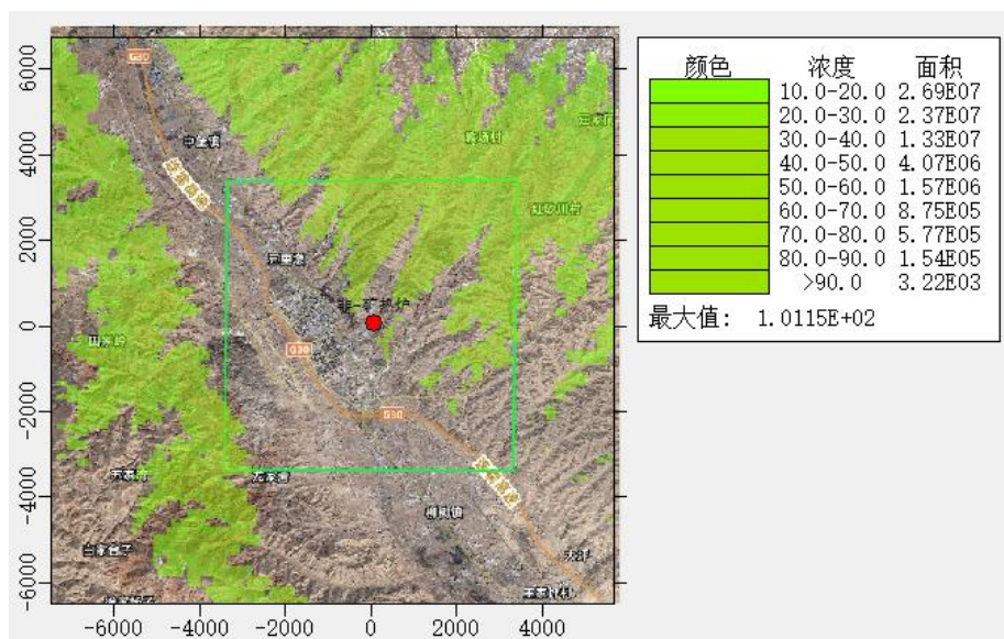
图 5.2-36 非正常工况 CO1 小时质量浓度预测图
