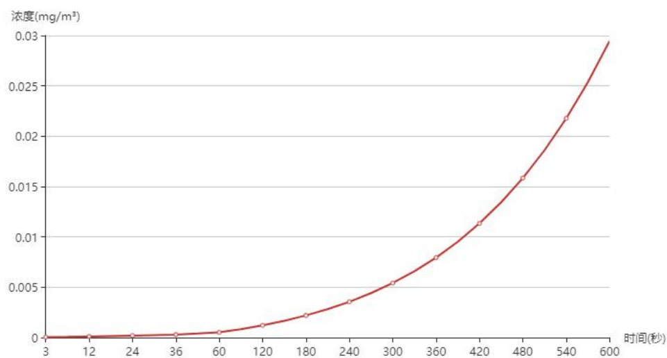
图 6.2-33 永登县职业中等专业学校浓度曲线图
