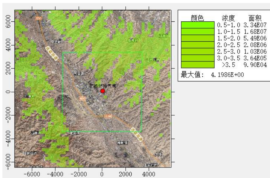
图 5.2-32 NO 2 24 小时质量浓度叠加预测图
