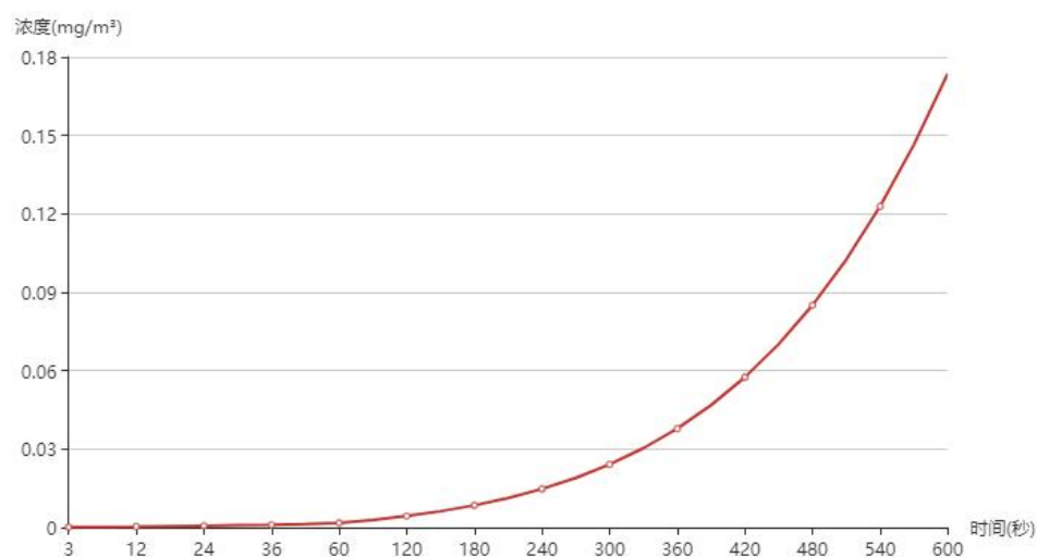
图 6.2-28 永登县中医医院浓度曲线图
