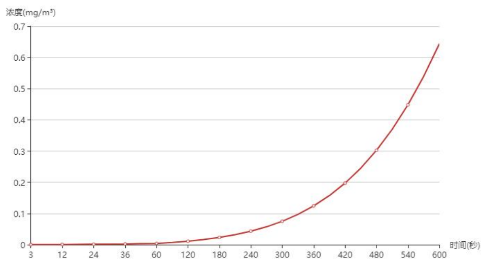
图 6.2-24 永登县应急管理局浓度曲线图
