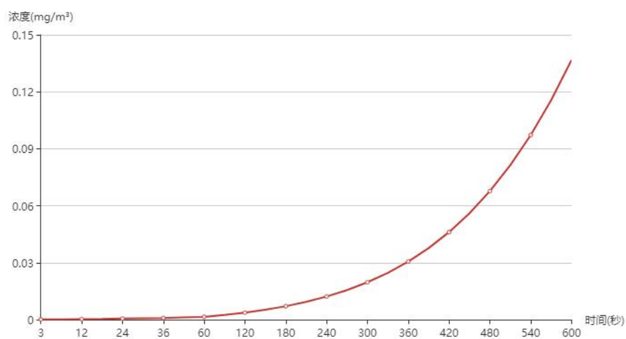
图 6.2-17 永登县公安局浓度曲线图
