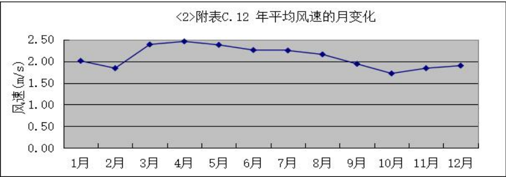
图 5.2-9 年平均风速月变化图
