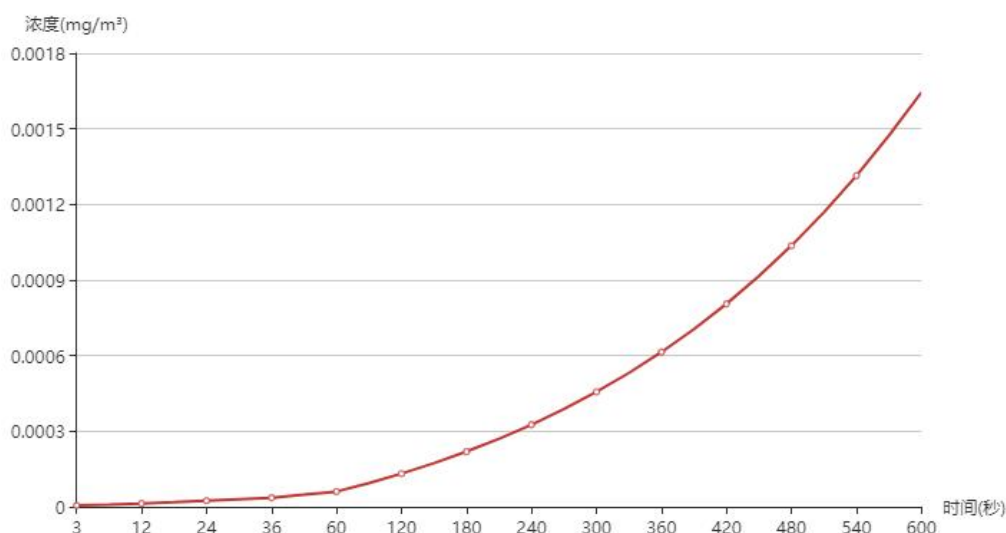
图 6.2-41 中堡镇汪家湾小学浓度曲线图
