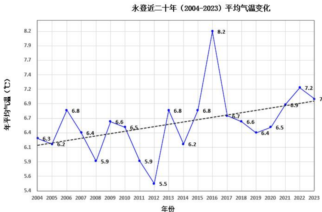
图 5.2-4 永登（2004-2023）年平均气温（单位：°C）
