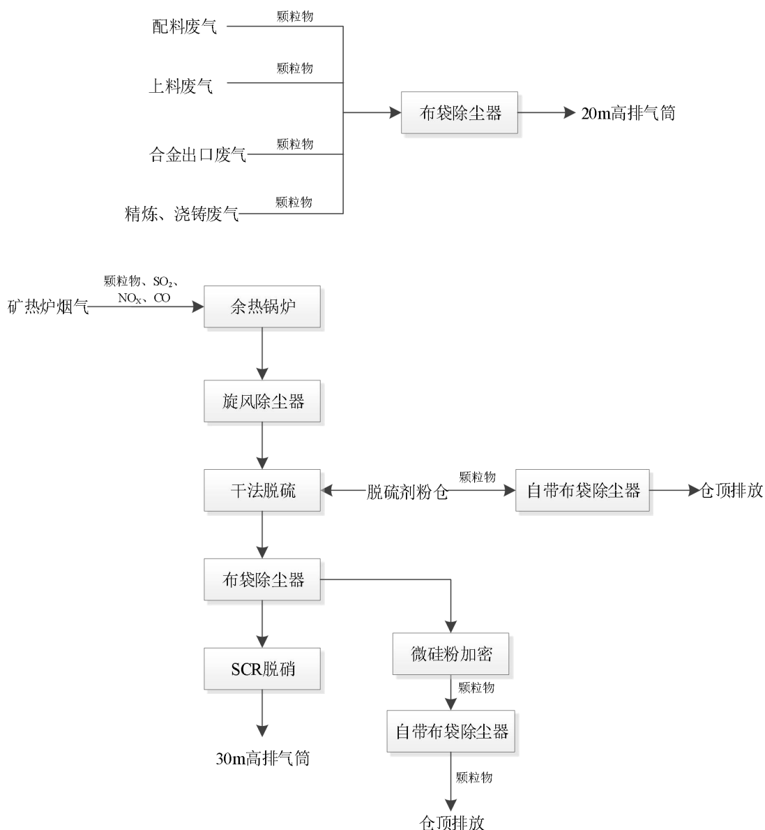
图 7.2-1 全厂废气处理措施图
