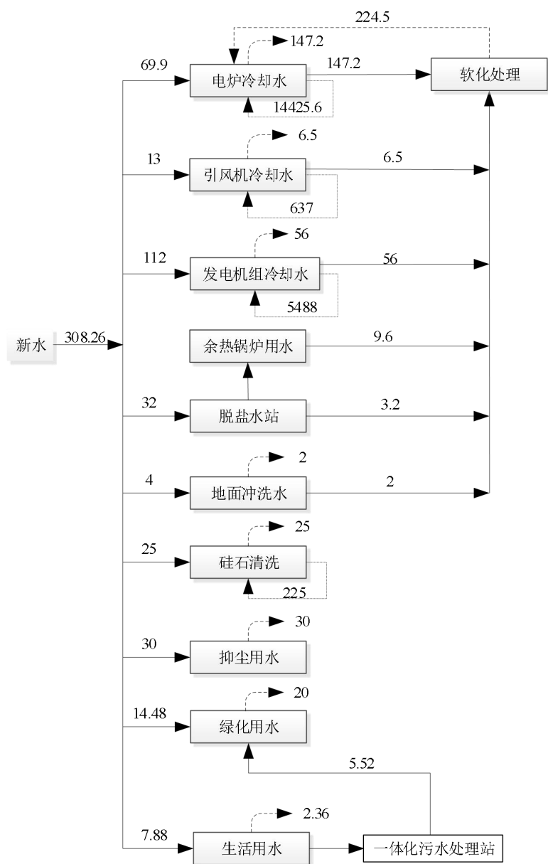
图 3.3-2 项目全厂水平衡图 单位: m³/d
